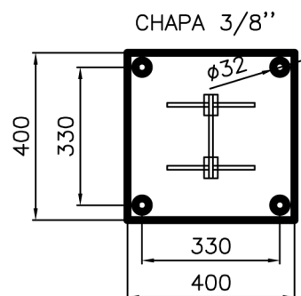
SAPATA FRONTAL ESCALA 1:10
