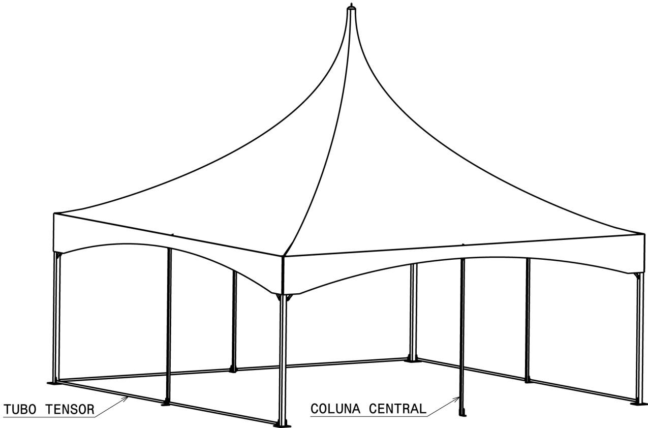
VISTA ISOMETRICA ESCALA: 1:90
