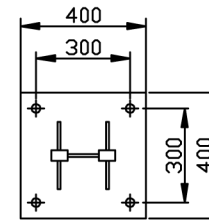
SAPATA ARTICULÁVEL TÍPICA GALPÃO DE 10M FURAÇÃO Ø32mm
