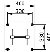
SAPATA ARTICULÁVEL TÍPICA GALPÃO DE 15 E 20M FURAÇÃO Ø32mm
